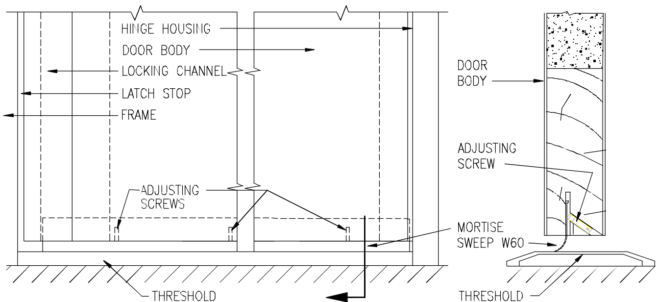
ELEVATION
