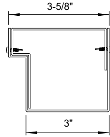
JAMB PROFILE
