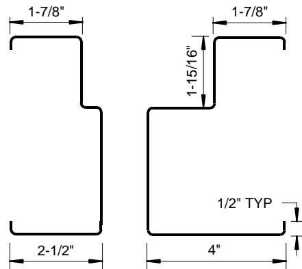
JAMB PROFILE
