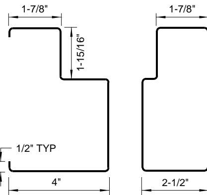
JAMB PROFILE
