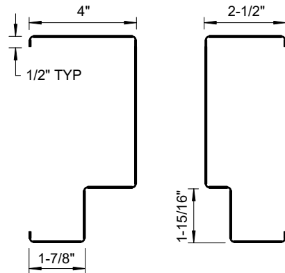
JAMB PROFILE
