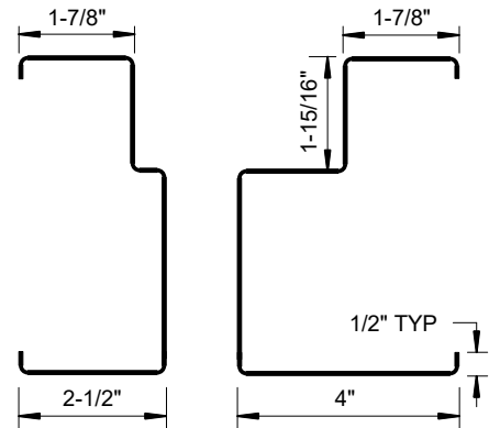
JAMB PROFILE
