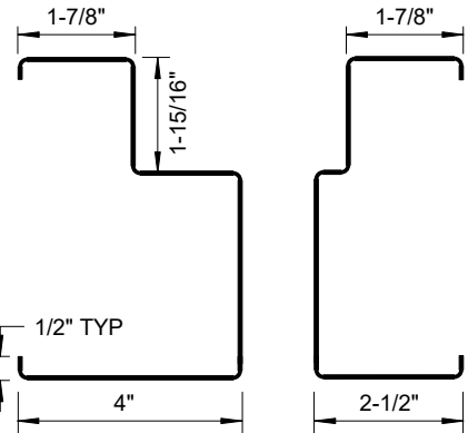
JAMB PROFILE
